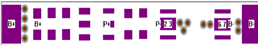
land pattern (焊盘示意图)
