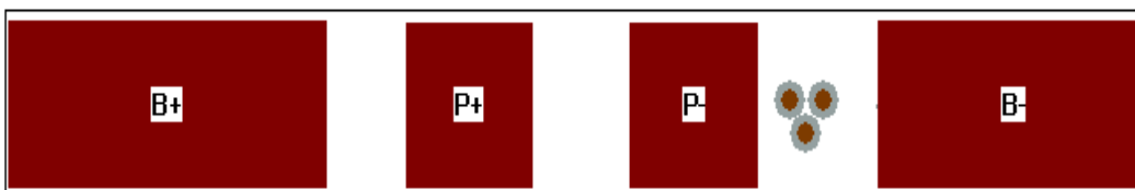
land pattern (焊盘示意图)
